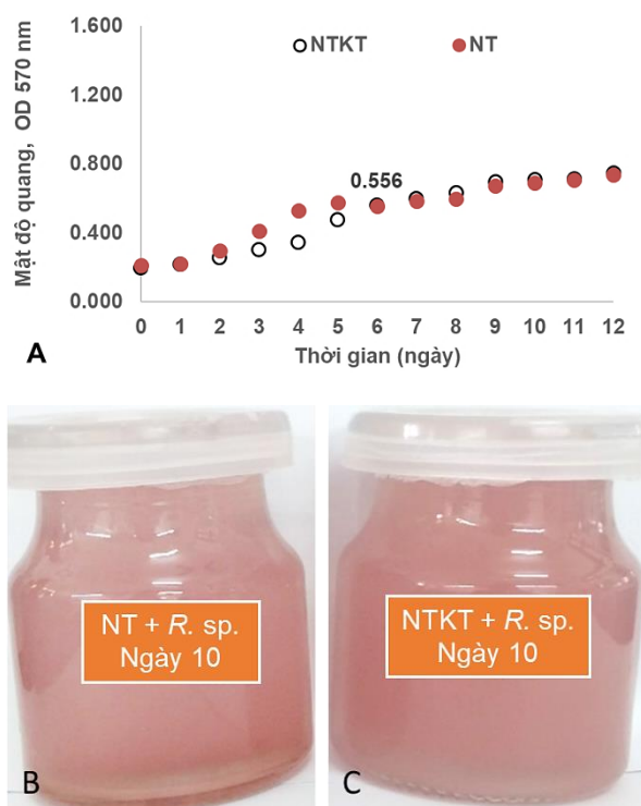
Hình 3. (A) Khả năng sinh trưởng của vi khuẩn Rhodopseudomonas sp. trong nước thải nuôi trồng thủy sản theo thời gian, (B) Ảnh chụp với mẫu không khử trùng (ngày 10) và (C) đã khử trùng (ngày 10)
