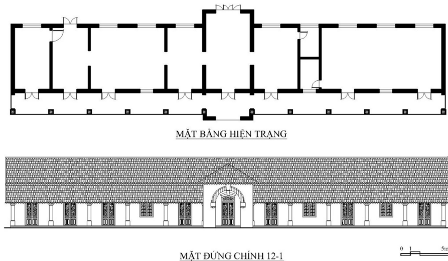
Hình 5: Bản vẽ mặt đứng và mặt bằng dãy nhà B, trường Cao đẳng công nghiệp (Nguồn: tác giả)
