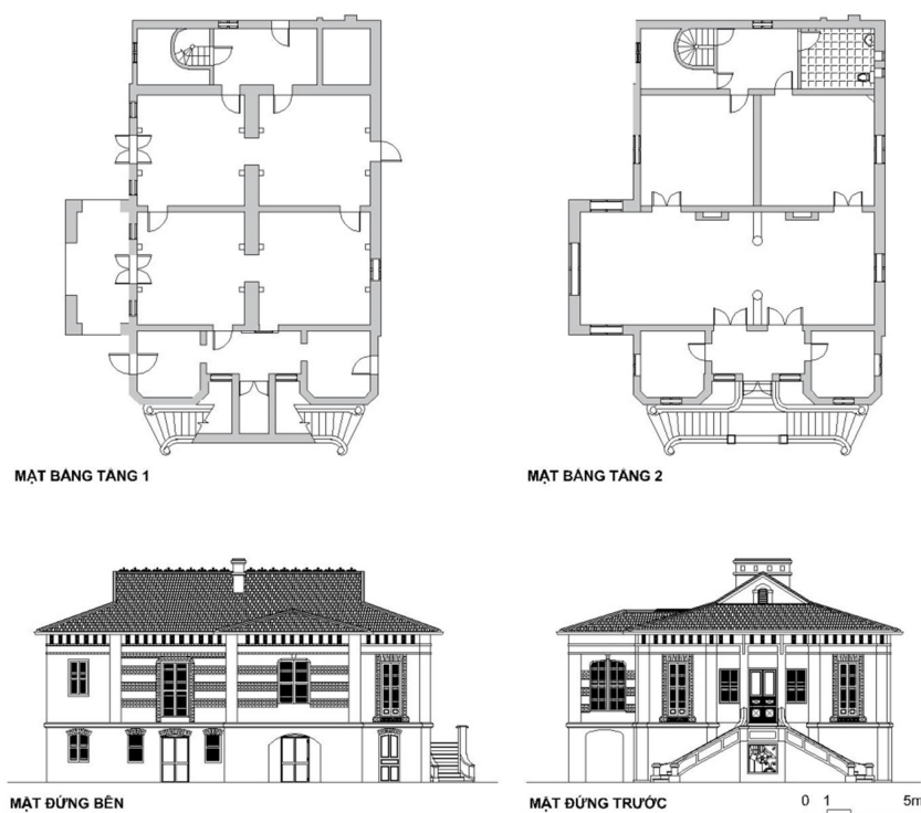
Hình 6. Bản vẽ mặt đứng và mặt bằng Liên hiệp các hội văn học nghệ thuật (Nguồn: tác giả)
