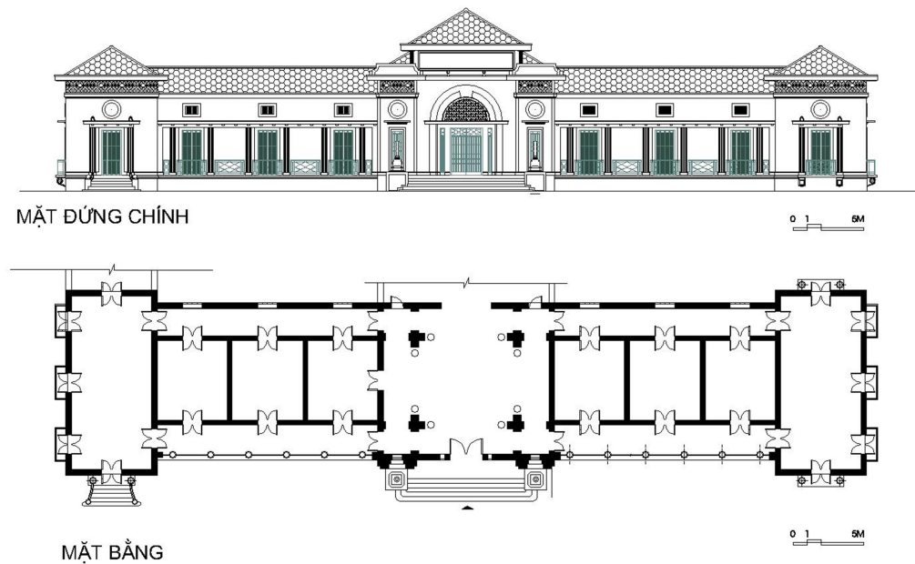
Hình 3. Bản vẽ mặt đứng và mặt bằng Trụ sở Đại học Huế (Nguồn: tác giả)
