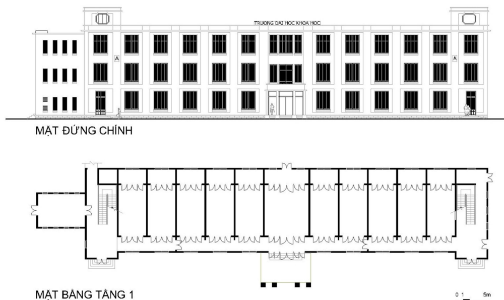
Hình 7: Bản vẽ mặt đứng và mặt bằng Trường Đại học Khoa học (Nguồn: tác giả)
